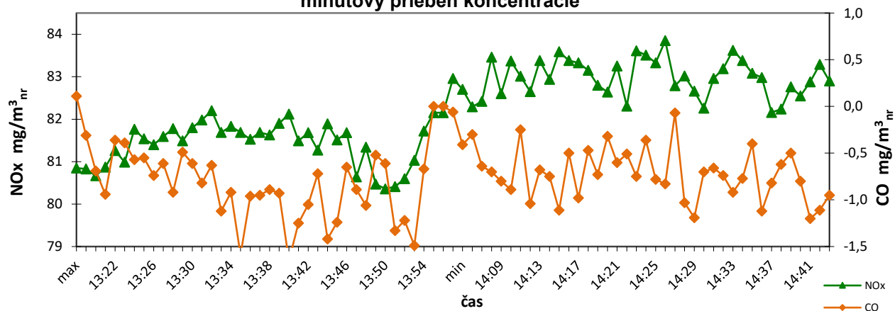
HK, Kotel K2 minútový priebeh koncentrácie
