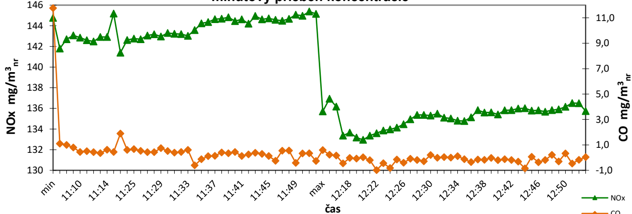
HK, Kotel K3 minútový priebeh koncentrácie
