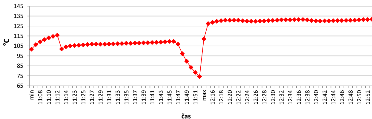
HK, K3 Minútový priebeh teploty odpadového plynu
