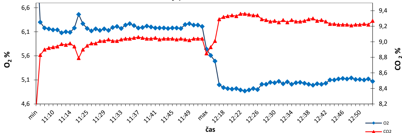
HK, Kotel K3 minútový priebeh koncentrácie
