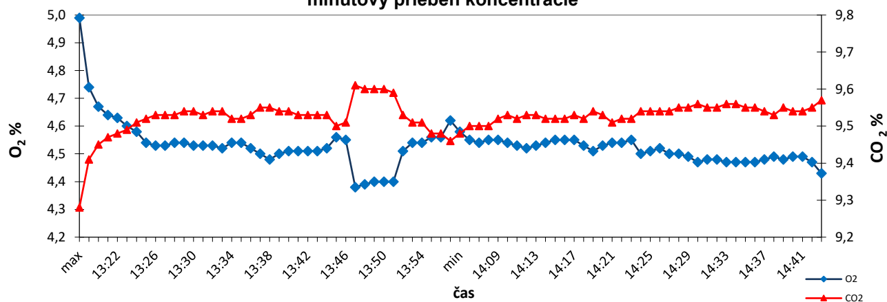
HK, Kotel K2 minútový priebeh koncentrácie
